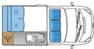
Ansicht Tag
